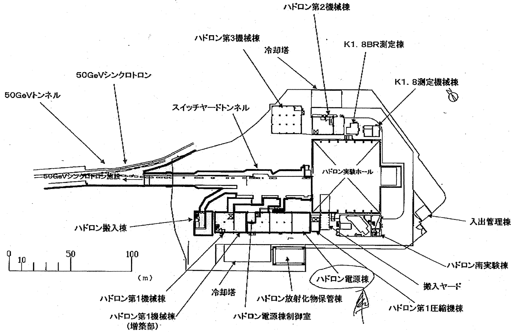
ハドロン実験施設平面図
