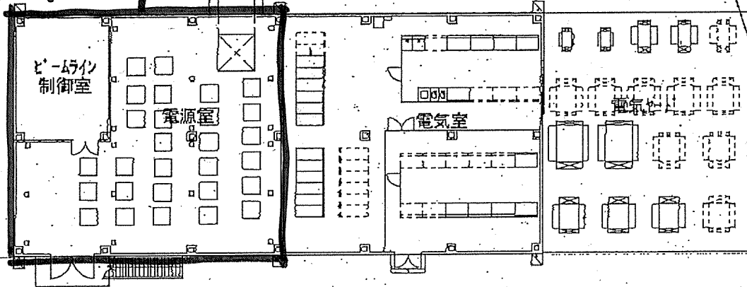
(a) 1階平面図
